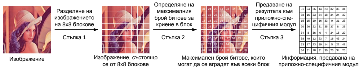
Фиг. 16: Базов модул – етап на подготовка ( PrepareToEncode )
