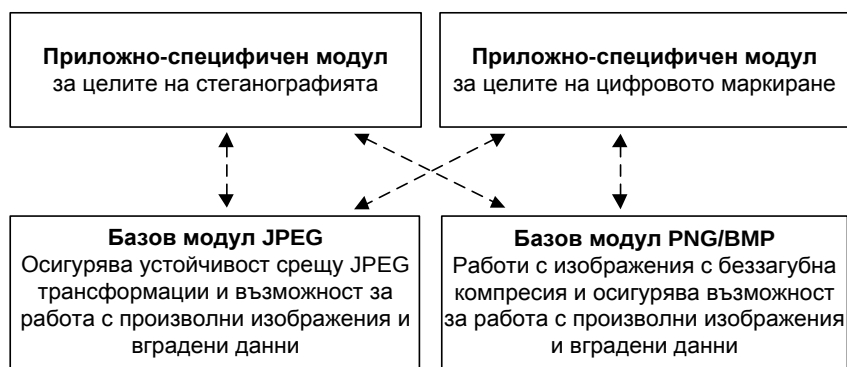
Фиг. 9: Модулен подход за криене на данни в мултимедия за целите на мрежови приложения
