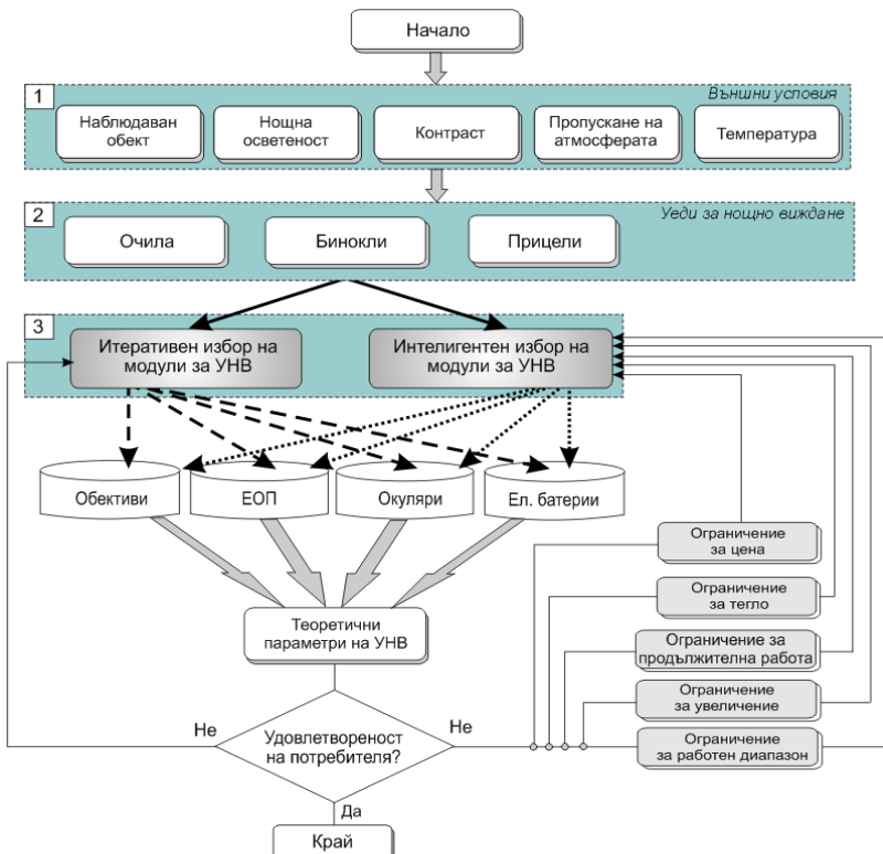
Фиг. 2.9. Блок-схема на предложения алгоритъм
