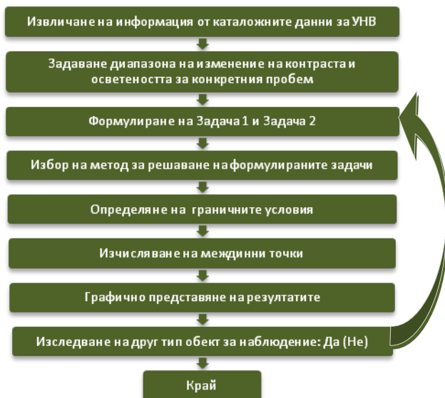
Фиг. 2.7. Етапи на предложената методология
