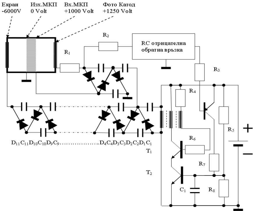
Фиг.3.13. Високоволтowo малогабаритно токозахранващо устройство
