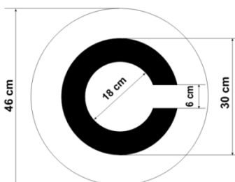
Фиг. 3.15. Размери на кръга на Ландолт
