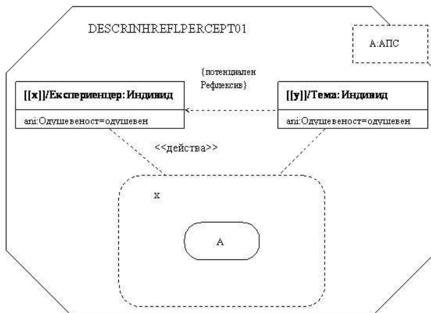
Фиг. 5. Рефлексивно значение - тип събитие възприемане
