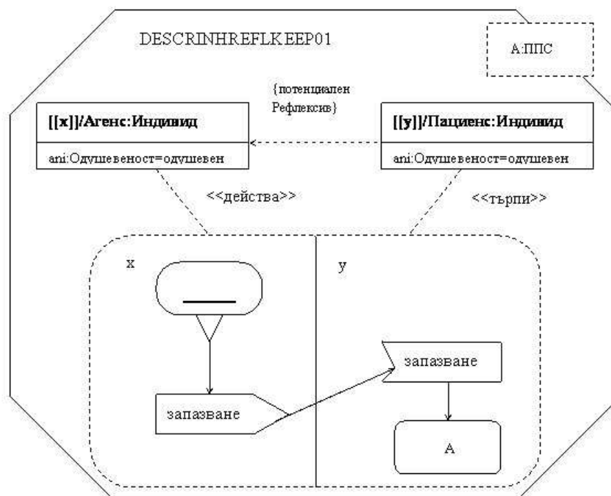
Фиг. 4. Рефлексивно значение със СИГНАЛ- запазване: вариант 1
