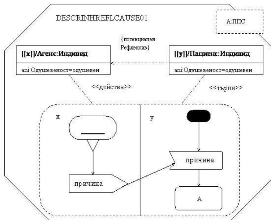
Фиг. 3. Рефлексивно значение със СИГНАЛ- причина: вариант 1
